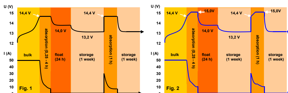
Krzywe ładowania: do osiągnięcia napięcia gazowania (wykres 1), po przekroczeniu napięcia gazowania (wykres 2)
